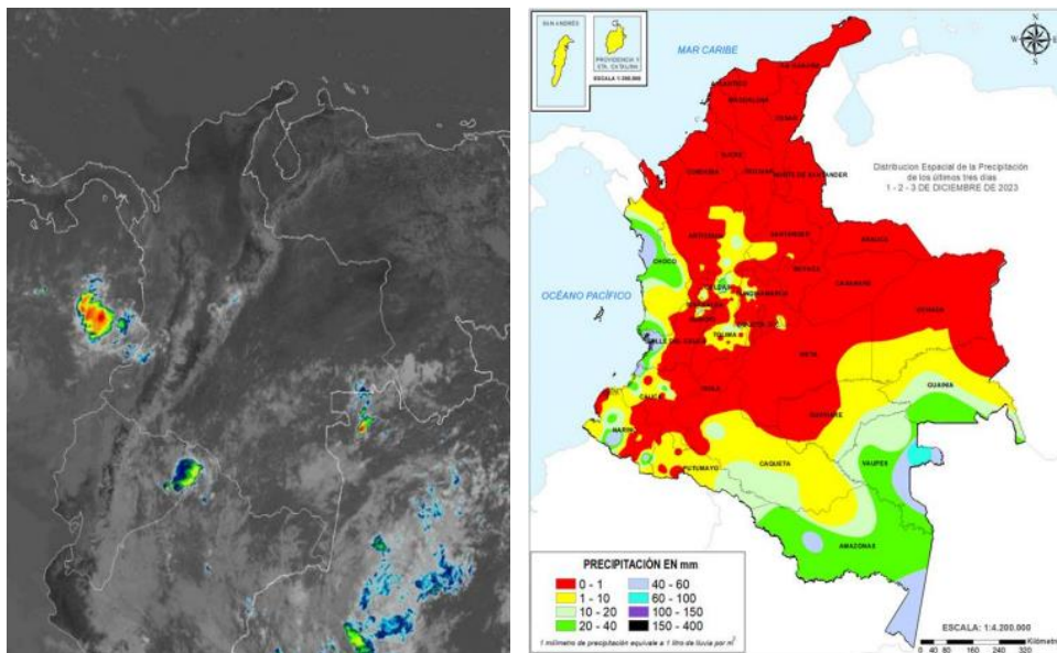
Imagen GOES East Canal Infrarrojo - Mapa de precipitación últimas 72 horas desde las 07:00 HLC del viernes 01, hasta las 07:00 HLC del lunes, 4 de diciembre de 2023
